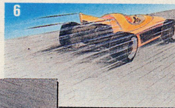
Bolide s'éloignant
