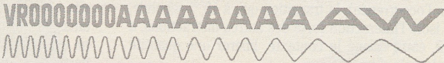
4 Bolide s'approchant
